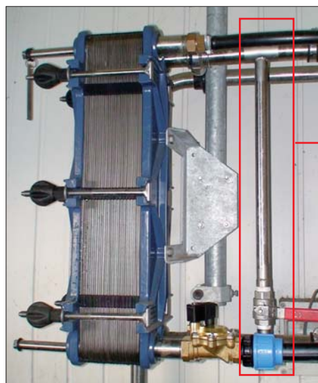
Système de nettoyage en « by-pass »
